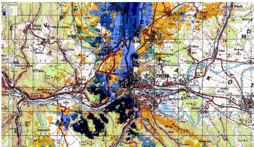
Obr. 4 – Vypočítané pokrytie územia z vysielača DVB-T na budove VÚS (TV kanál K27, ERP_{max} = 200\text{ W} )
